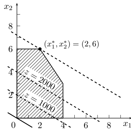
repérage de la solution graphique
