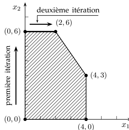
le chemin suivi par l'algorithme du simplexe
