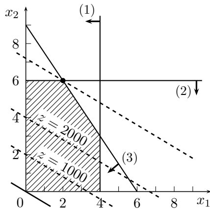
droite d'isoprofit la plus élevée
